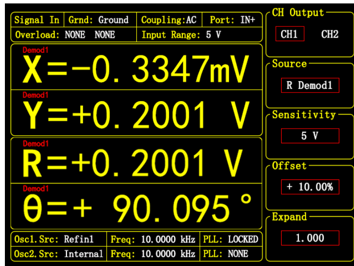
图 67. &lt;Offset&amp;Expand&gt; 界面
