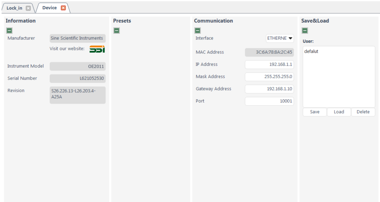
图 83. [SYSTEM] 的配置区域
