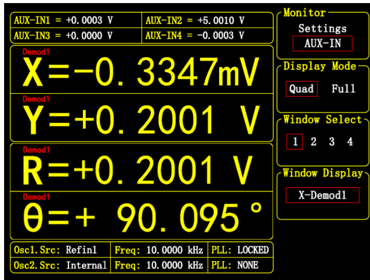
图 57. <AUX-IN> 界面
