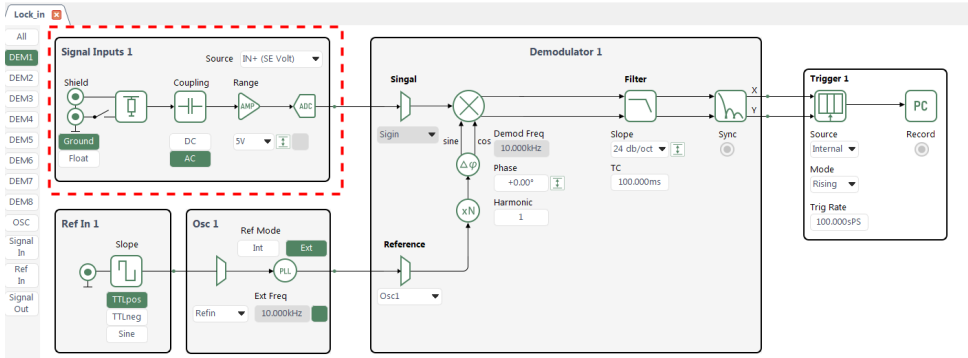
图 41. [SIGNAL INPUT] 的配置区域
