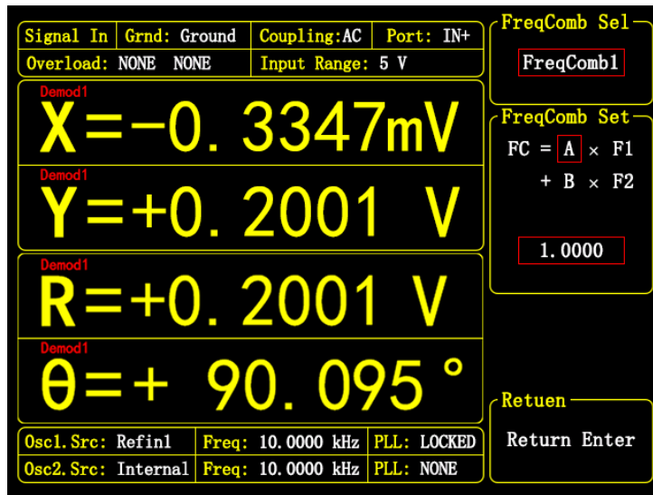
图 53. <FreqComb> 二级菜单设置界面
