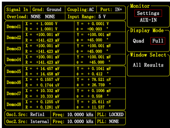
图 58. <Full> 显示模式
