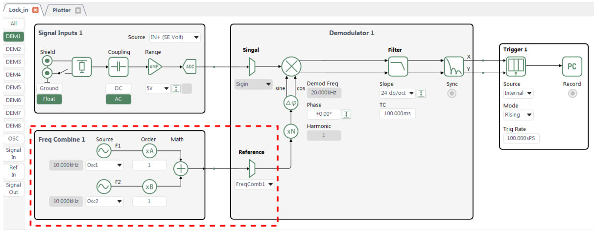
图 55. [DEM0D REF] 的 FreqComb 公式配置区域
