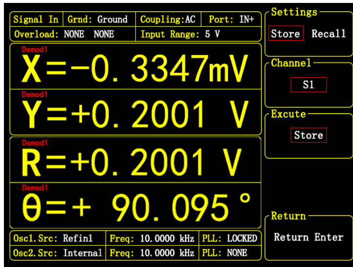
图 81. [Store/Recall] 子菜单
