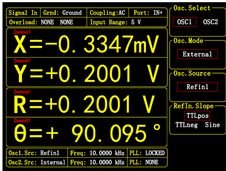
图 42. [OSC REF] 子菜单-<External>
