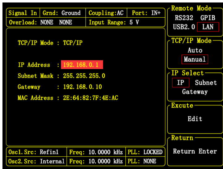
图 80. &lt;Manual&gt; 模式修改中
