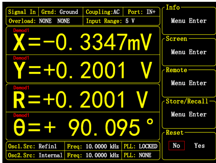
图 69. [SYSTEM] 子菜单
