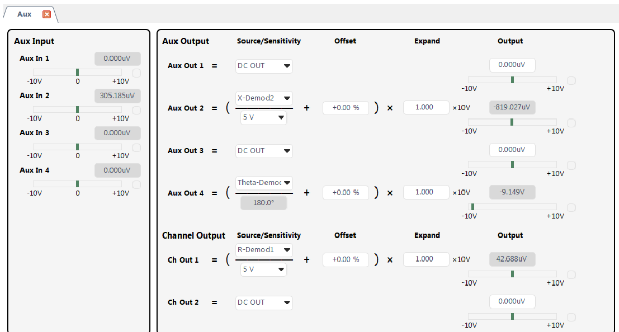
图 68. [CHOUT AUXOUT] 的配置区域
