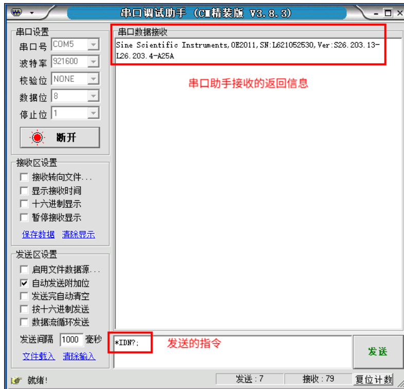
图 110. ASCII 码形式发送和接收指令
