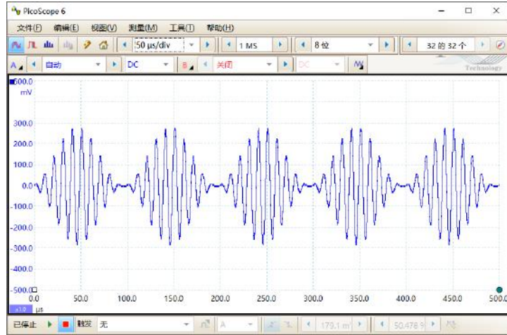
图82. AM 调制信号的波形
