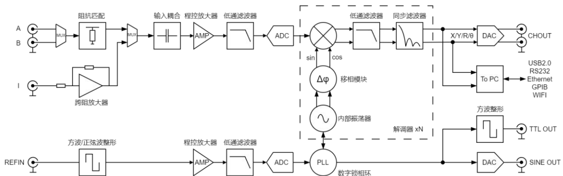
图6. OE2011/OE2021 原理框图
